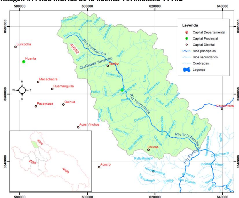
Imagen 07: Red hídrica de la Cuenca Torobamba 49982
