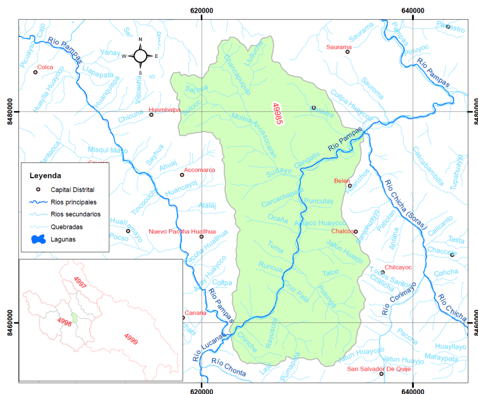
Imagen 04: Red hídrica de la Intercuenca del río Pampas ( 49985 )
