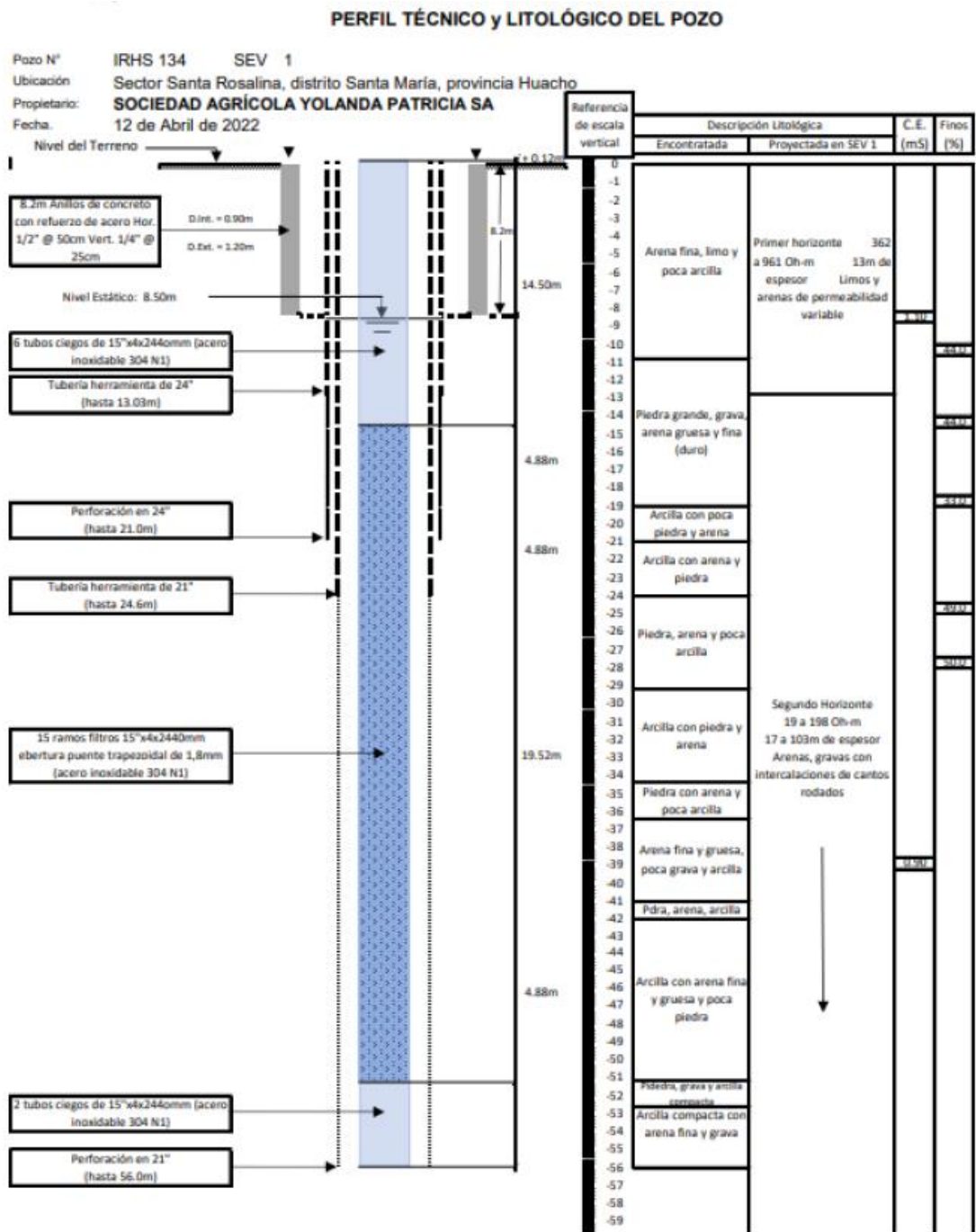
Imagen N° 2. Perfil del pozo.
